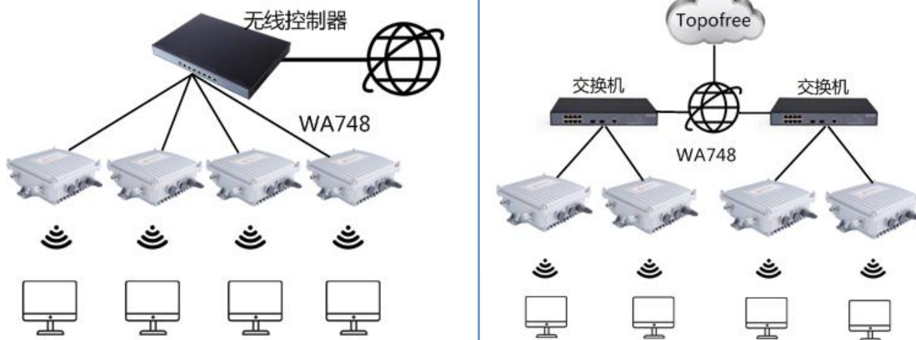
集中管理（本地AC与敦崇云平台）
